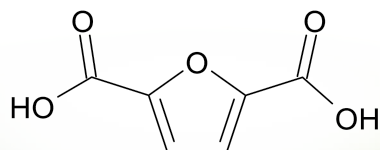
●2,5-フランジカルボン酸
