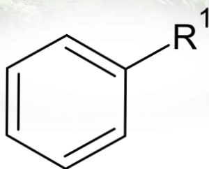
●芳香族化合物
